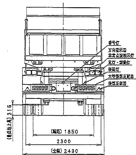
東邦TU30D7C2S型 ダンプセミトレーラ外觀四面図
