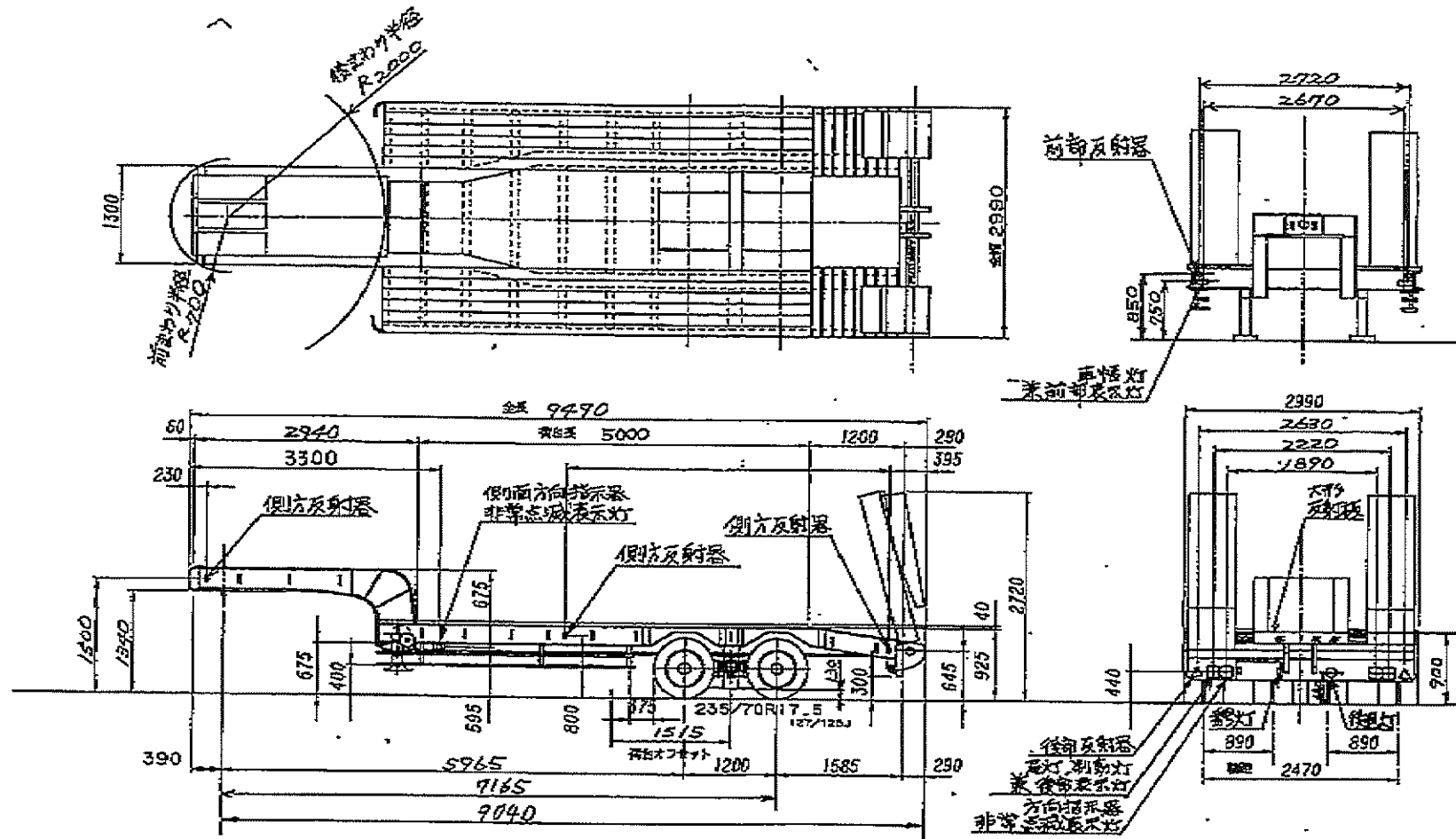
トレーラーモービル PLR430AG型 外観四面図
