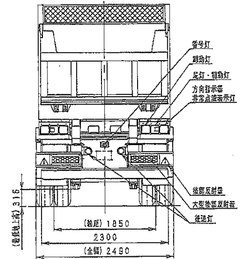
東邦TF36H2C3改型 ダンプセミトレーラ外觀四面図
